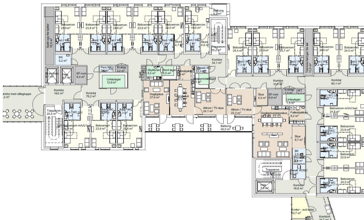
Sykehjemsavdelinger 3. etg.
