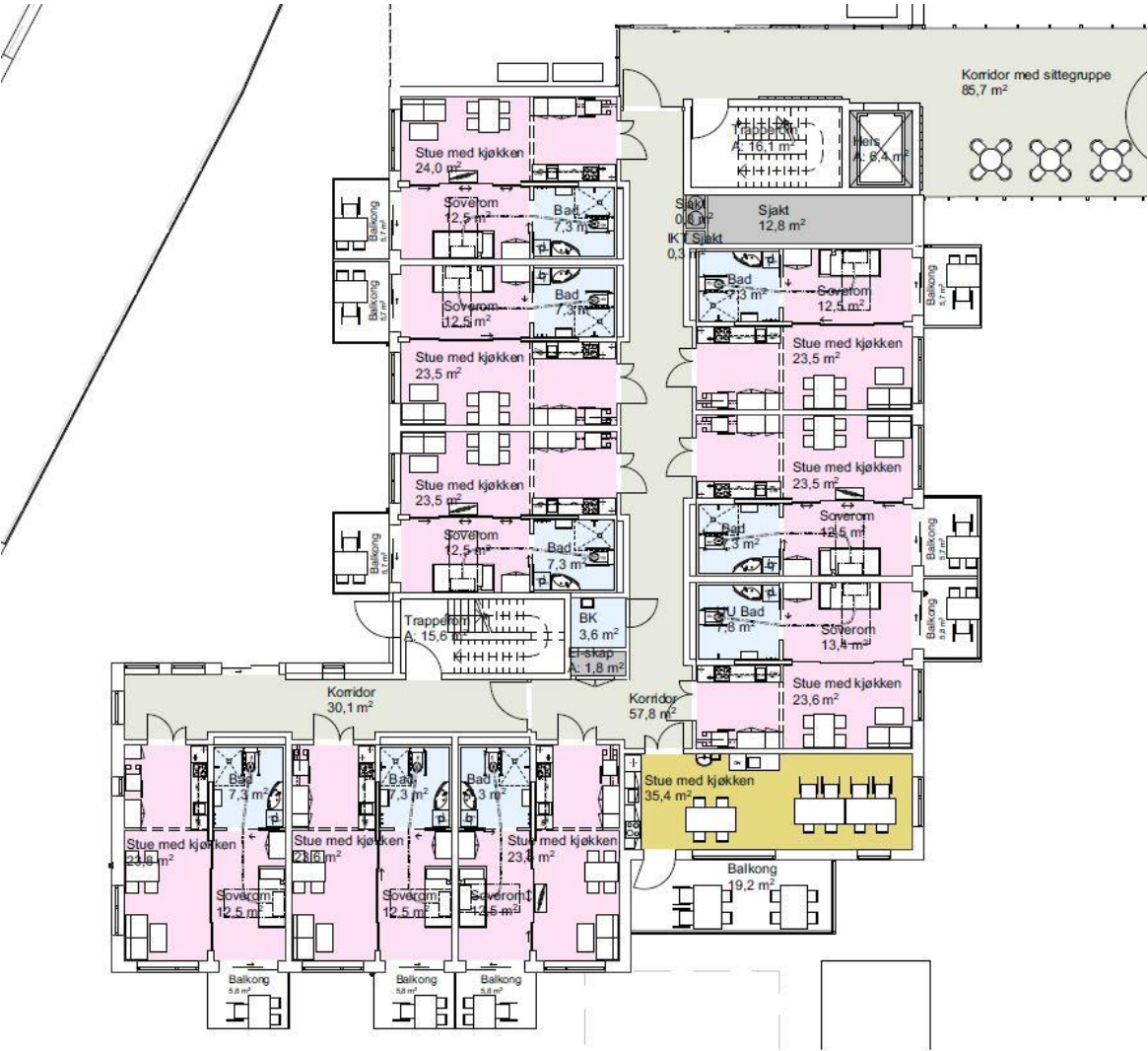
Omsorg+-bolig 2. etg.
