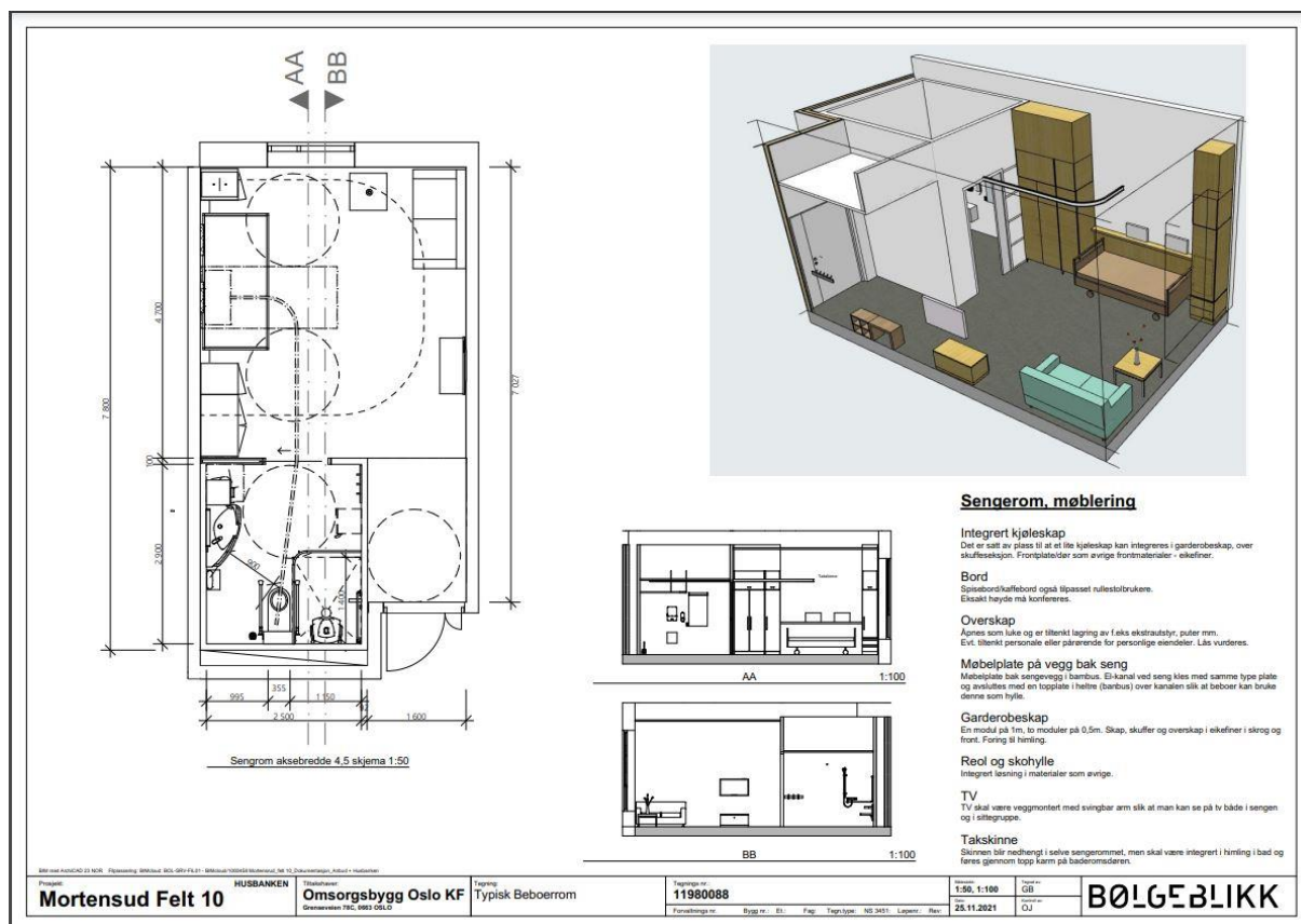
Beboerrom sykehjem
