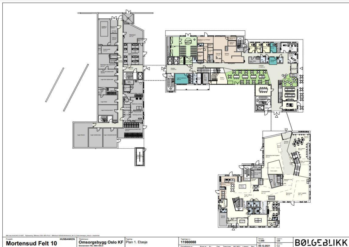
Plantegning 1. etg.
